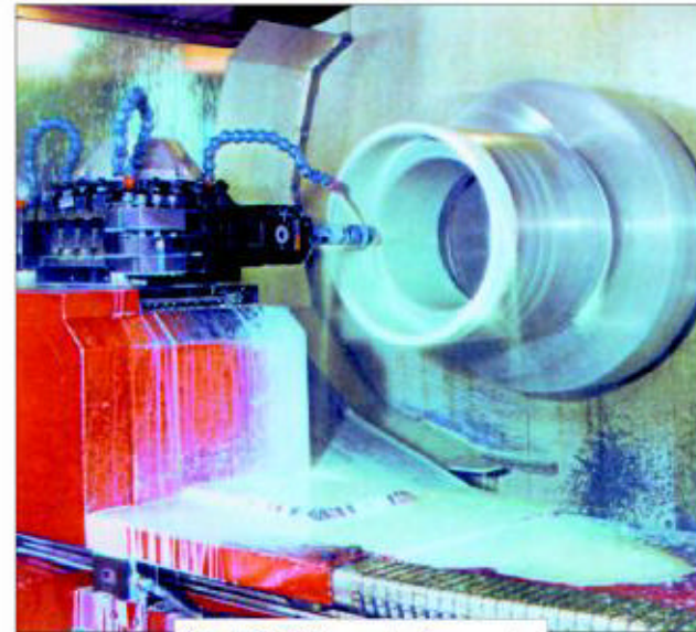
Tornio GIANA a controllo numerico GIANA CNC lathe
